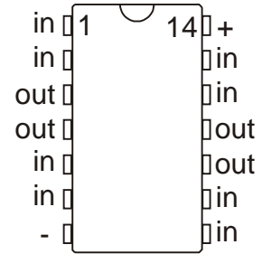
4093
