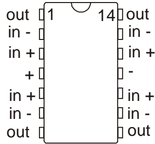
TL084
